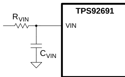
Figure 28. VIN Filter
