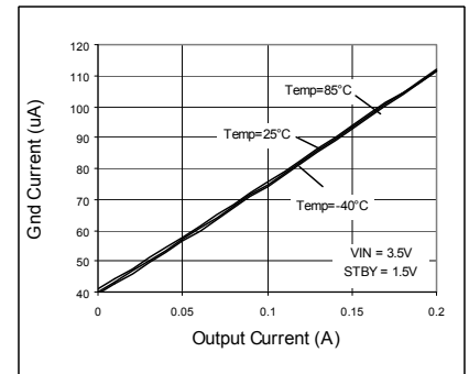
Fig. 71. IOOUT - IGND
