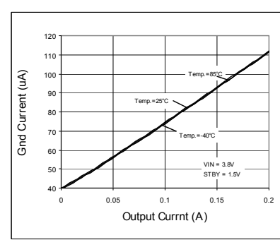
Fig. 16. IOU - IGND
