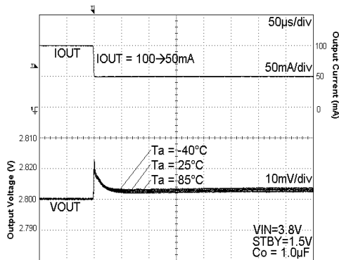
Fig. 26. Load Response
