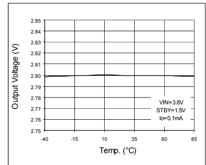
Fig. 19. VOUT vs. Temp
