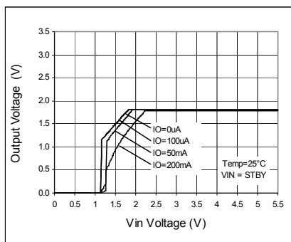
Fig. 37. Output Voltage
