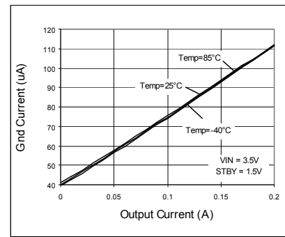
Fig. 42. IOUT - IGND
