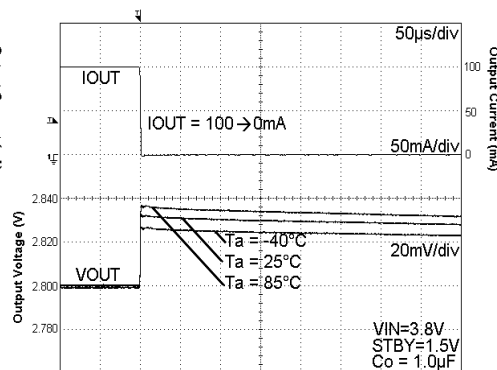
Fig. 24. Load Response
