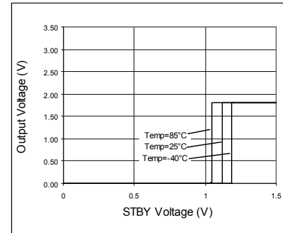
Fig. 45. STBY Threshold
