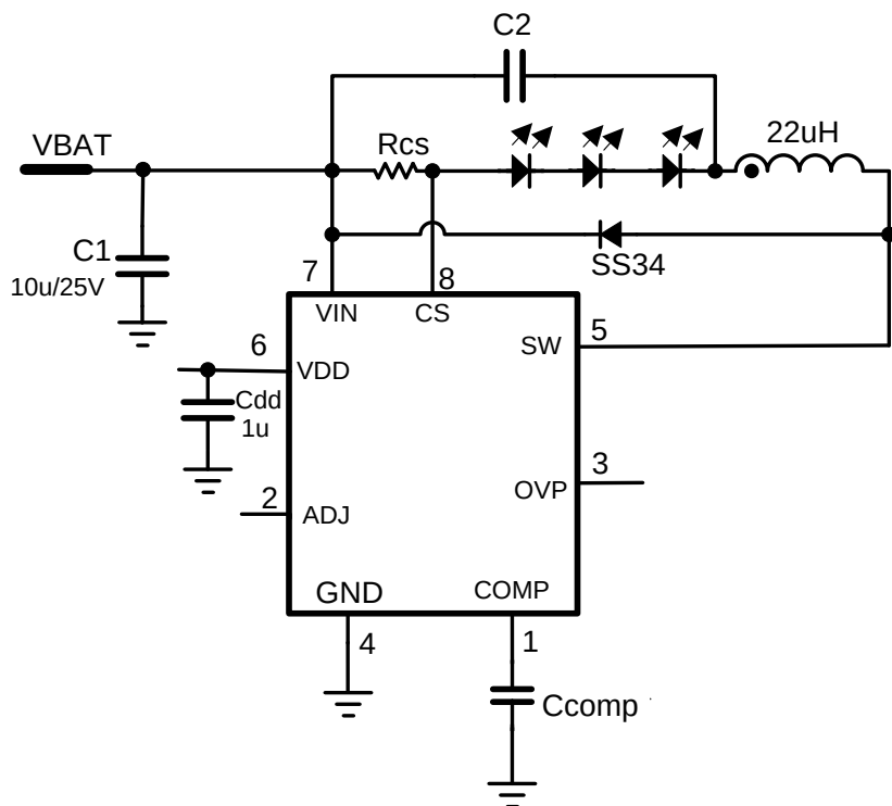
图 4、BUCK 应用 V_{BAT} > V_{LED}
