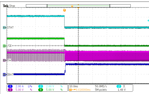
图 9-10. Charge Enable
