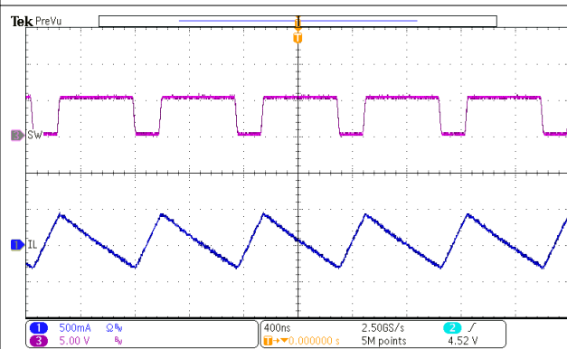
图 9-12. OTG Switching
