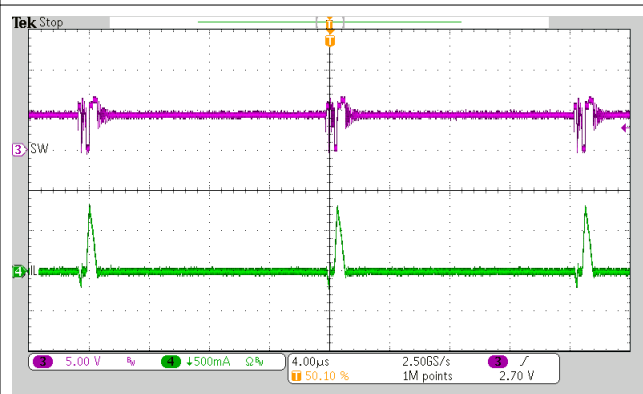
图 9-10. Charge Enable
