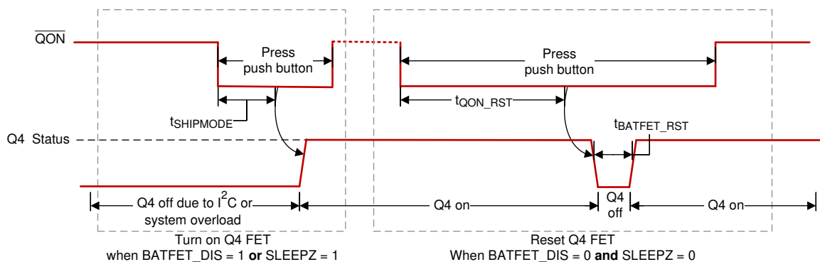
图 8-10. \overline{QON} Timing
