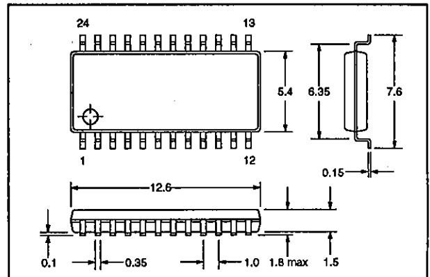
3112-MFP24S (LA2230M)
