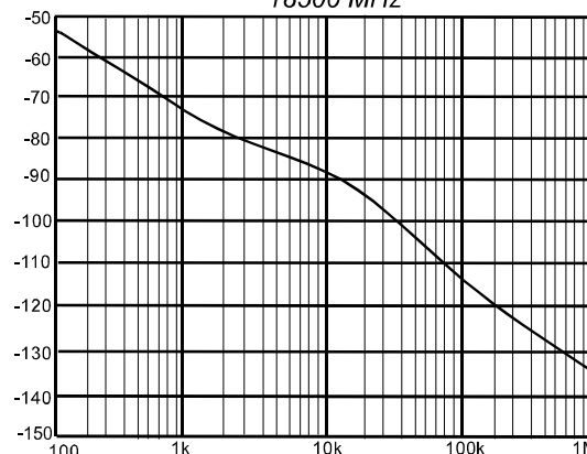
Phase Noise (dBc/Hz) 18500 MHz
