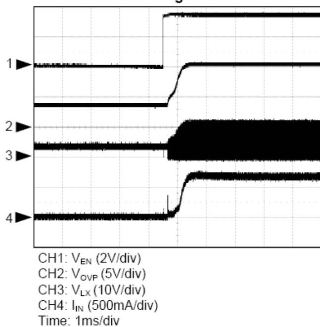
EN Goes High- Enable
