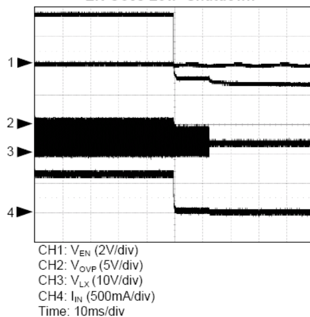
EN Goes Low- Shutdown
