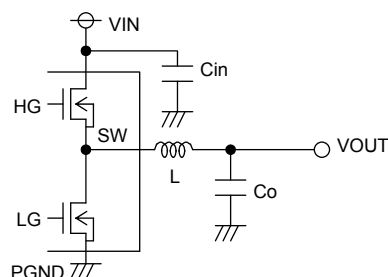
Input Capacitor
