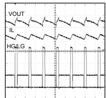
Fig.21 SLLM Mode ( I_{OUT}=1A )
