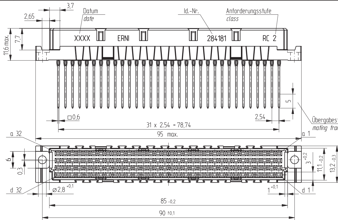
Bestückungsplan / contact layout
