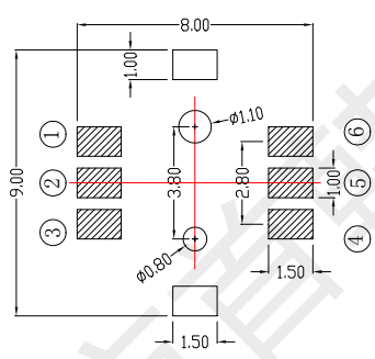
印制板安装孔图
