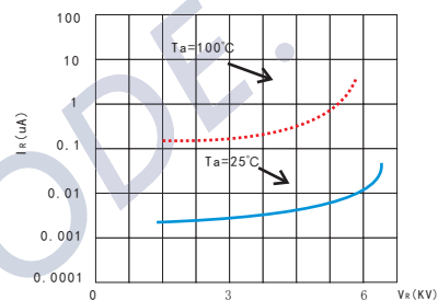
反向特性曲线(2CL70) Reverse Characteristics
