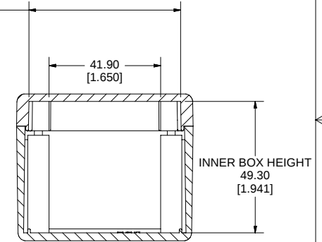
SECTION D-D SCALE 1 : 1
