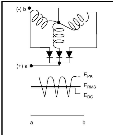
Fig. 4 : Half wave
