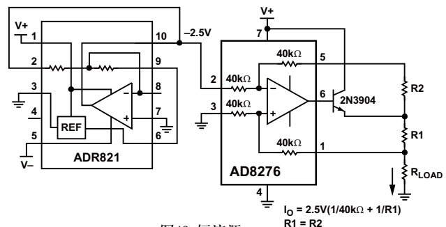
图49. 恒流源
