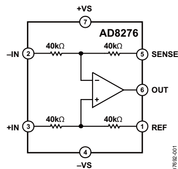
图1. AD8276
