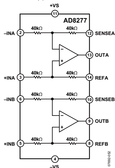
图2. AD8277
