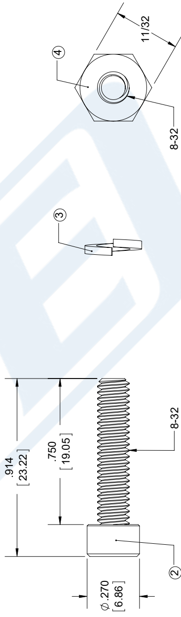
SECTION A-A
