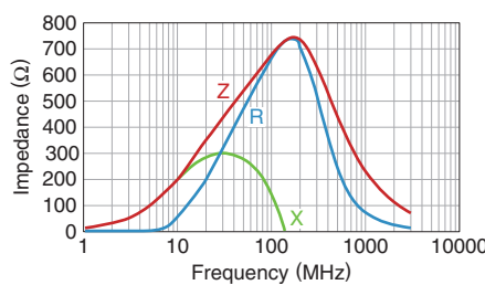
MPZ1608Y600BTA00
