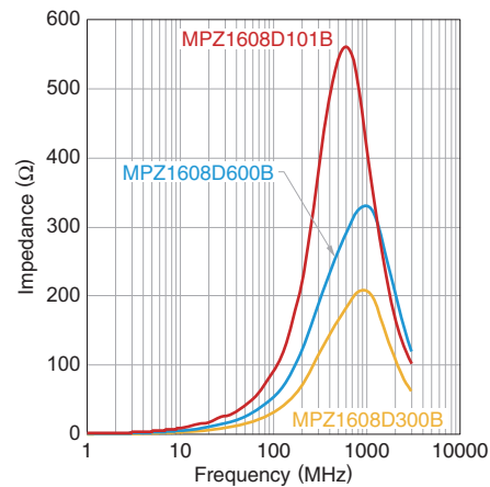
MPZ1608D系列
