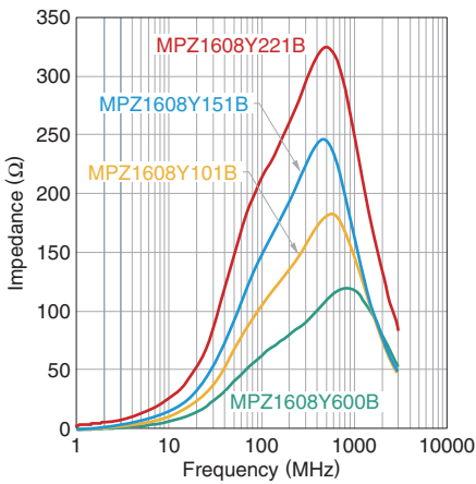
MPZ1608Y系列
