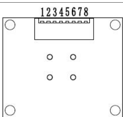
图 2： 模组引脚图
