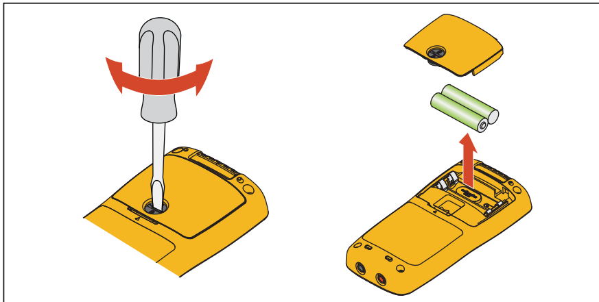
图 5. 更换电池
