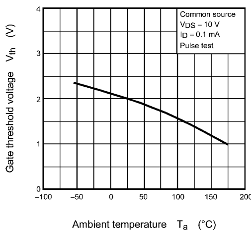
Fig. 8.9 V_{th} - T_a
