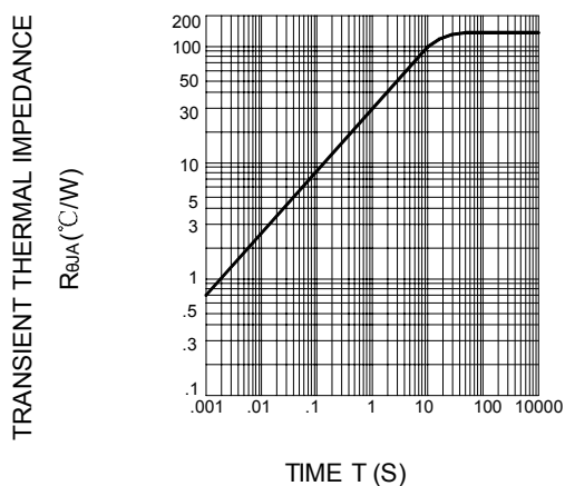
FIG.4 -- R_{\theta JA} - T
