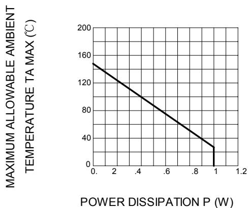
FIG.4 -- R_{\theta JA} - T
