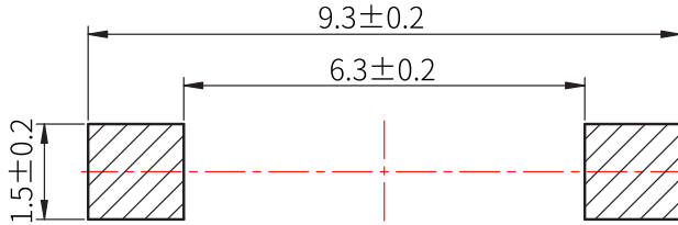
RECOMMENDED P.C.B LAYOUT 安装尺寸图
