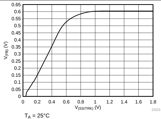
图 23. V_{(FB)} vs V_{(SS/TRK)}
