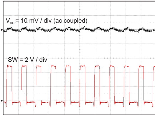
图 59. V_{DD} Output Ripple
