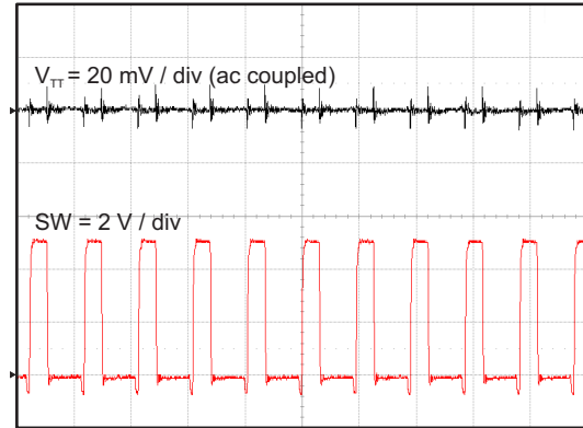
图 60. V_{TT} Output Ripple
