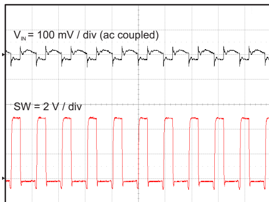
图 61. Input Ripple
