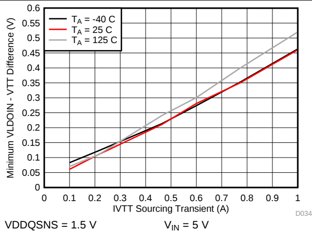
图 33. VTT Dropout
