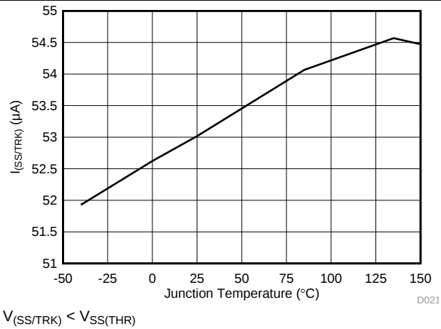
图 21. I_{(SS/TRK)} vs Temperature
