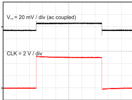
图 63. V_{TT} Output Transient Response
