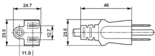
NEMA5-15
