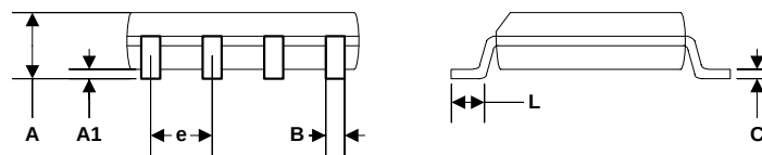
SOP8
