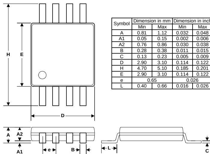
MSOP8
