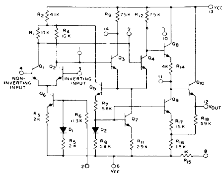
CA3029A, CA3030A
