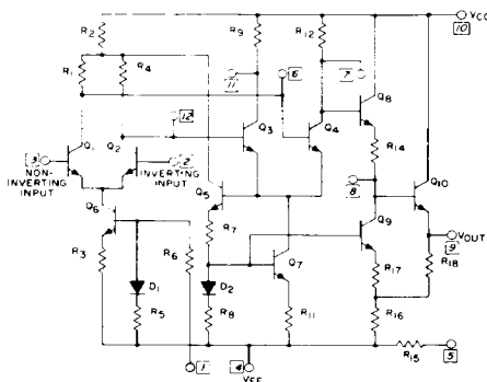
CA3010A, CA3015A
