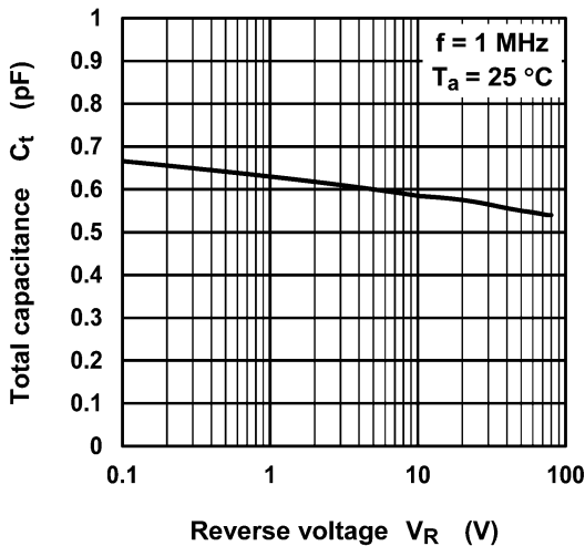
Fig. 7.3 C_t - V_R
