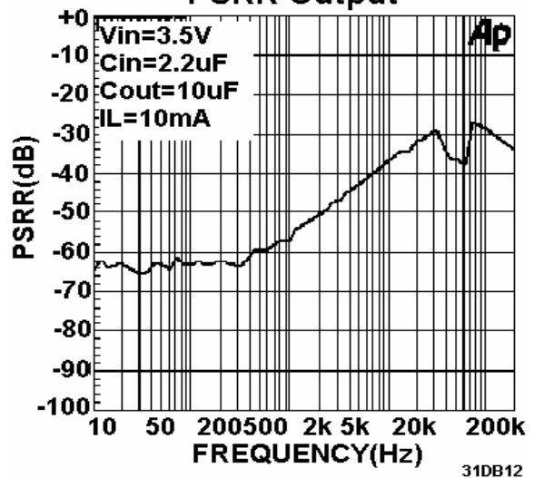
PSRR Output
