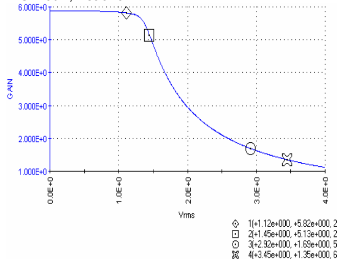
IAC=20uA, Veao=6V
