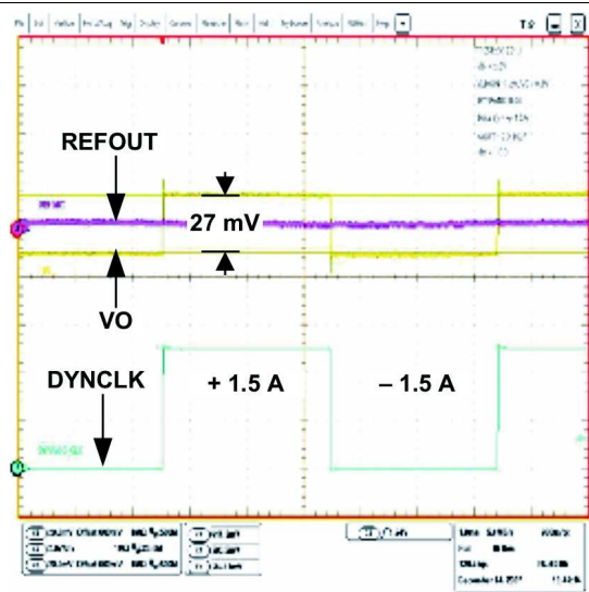
图 25. Transient Waveform
