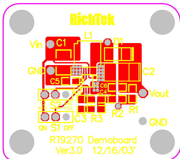
Top Side
