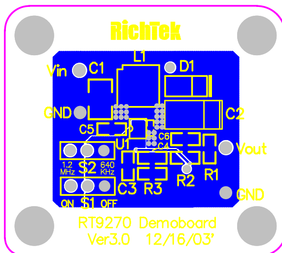
Bottom Side
