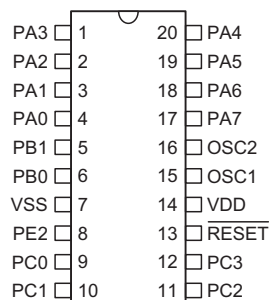
HT82K68E-L/HT82K68A-L —20 SOP-A
