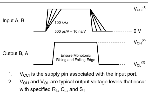
图 7-3. Input Transition Rise or Fall Rate
