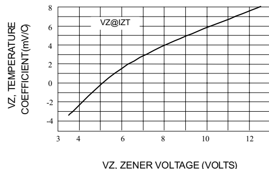
Fig. 2-ZENER VOLTAGE- 5.1 TO 12 VOLTS
