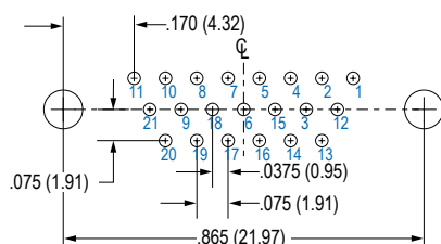
21 SOCKET
