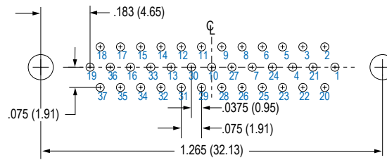
37 SOCKET
