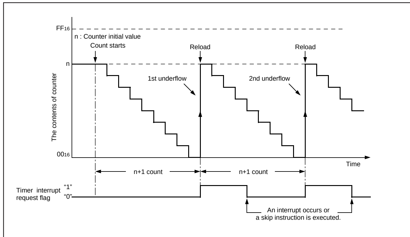
Fig. 18 Auto-reload function
