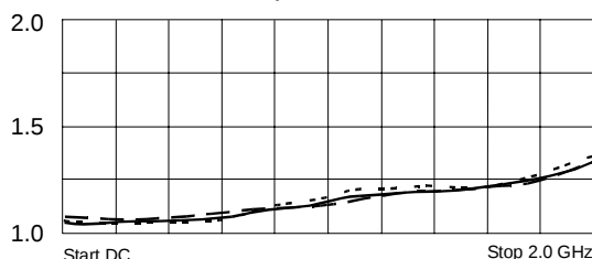
Input VSWR
