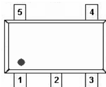
SOT23-5L/TSOT23-5L (Top View)
