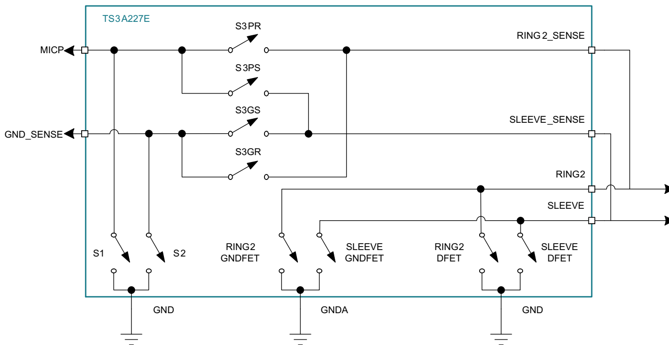
图 26. Switch Diagram
