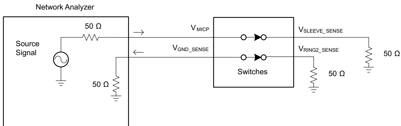
图 13. Channel Separation
