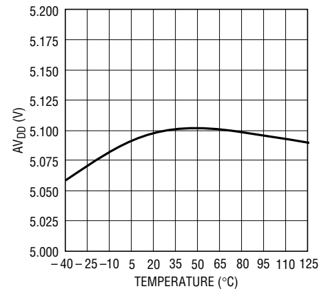
AV DD vs Temperature Figure 1 Circuit, 1mA Load
