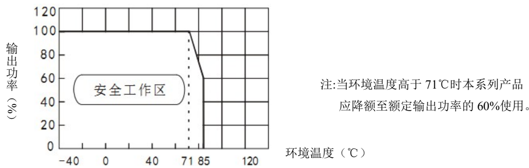
温度曲线图
