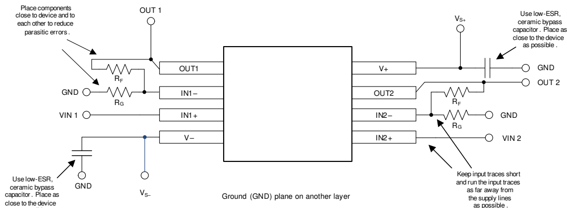
图 10-2. 布局示例
