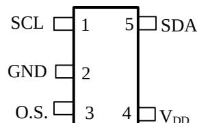
DS1775R SOT23-5
