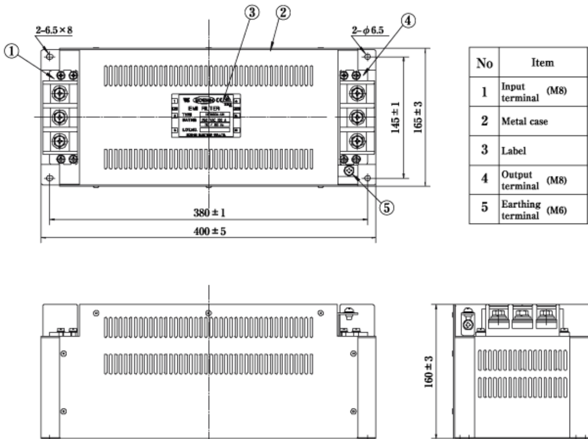
fig. 3 (100A)
