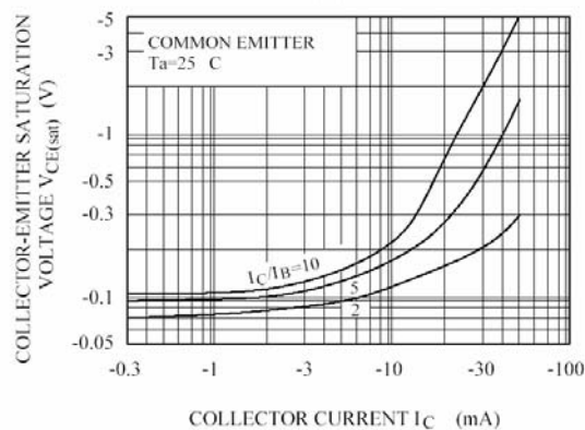
V_{CE(sat)} - I_C
