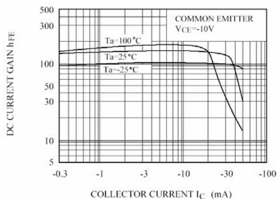
h_{FE} - I_C
