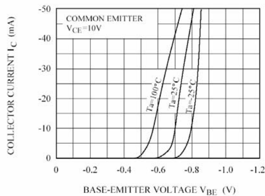
I_C - V_{BE}
