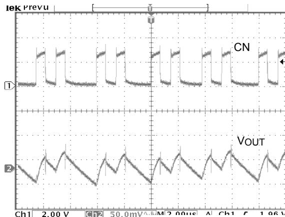
Fig. 14 Output Ripple
