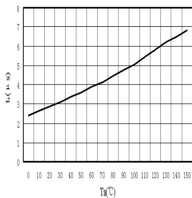
t_s-T_a
