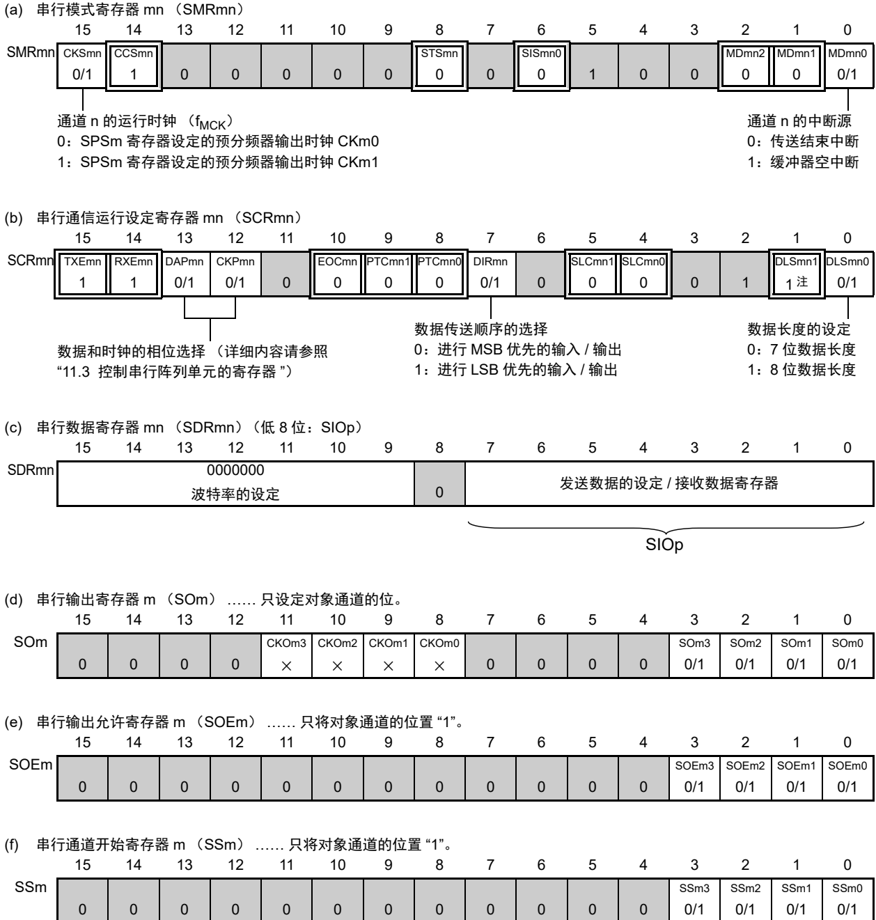
图 11-62 3 线串行 I/O (CSI00、CSI11、CSI20) 从属发送和接收时的寄存器设定内容例子
