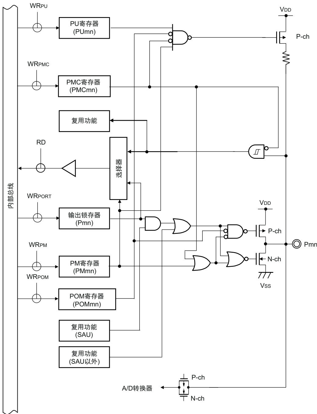
图 2-8 引脚类型 7-3-2 的引脚框图
