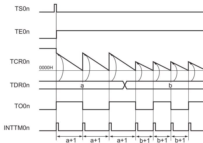
图 6-38 作为间隔定时器 / 方波输出运行的基本时序例子 (MD0n=1)
