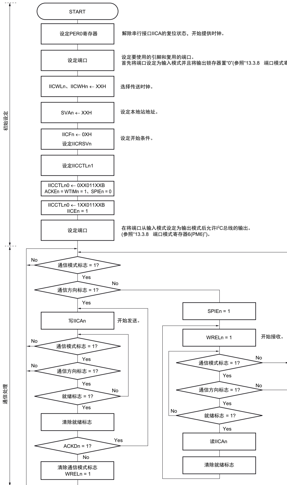
图 12-30 从属运行步骤 (1)
