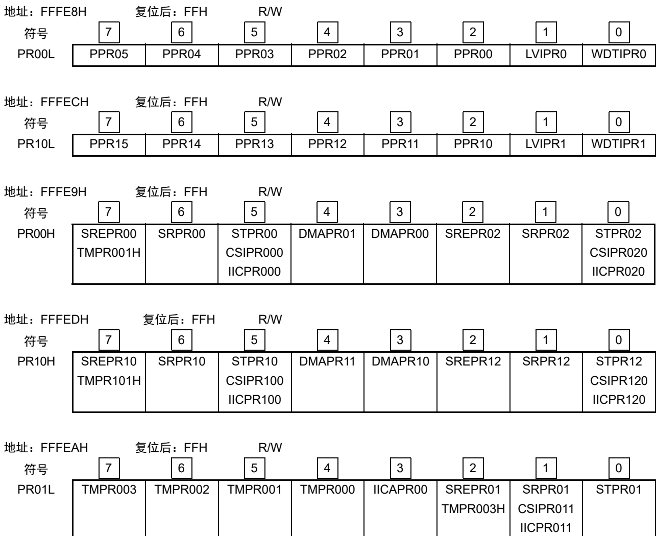
图 15-4 优先级指定标志寄存器 (PR00L、PR00H、PR01L、PR01H、PR02L、PR02H、PR10L、PR10H、PR11L、PR11H、PR12L、PR12H) 的格式 (1/2)
