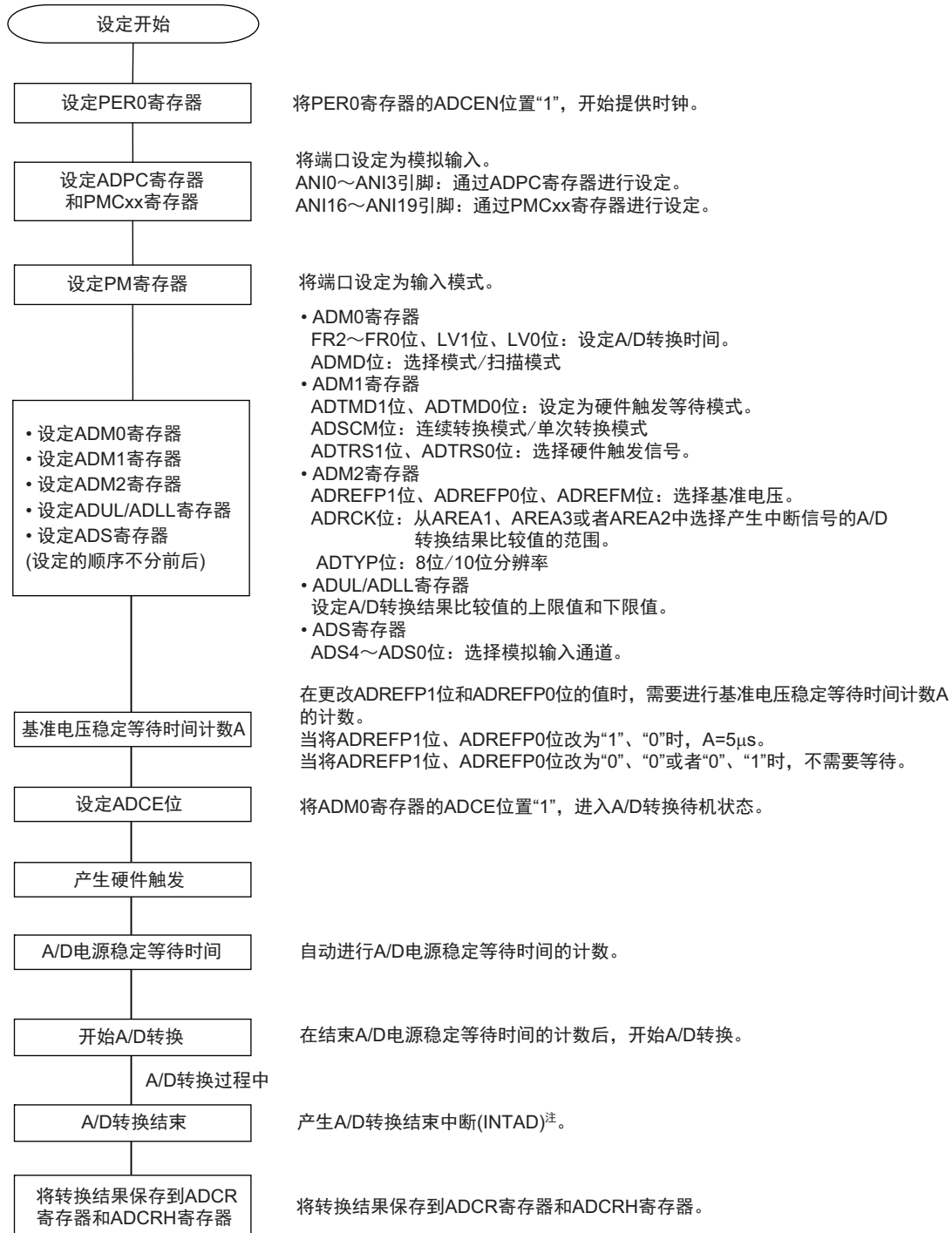
图 10-31 硬件触发等待模式的设定
