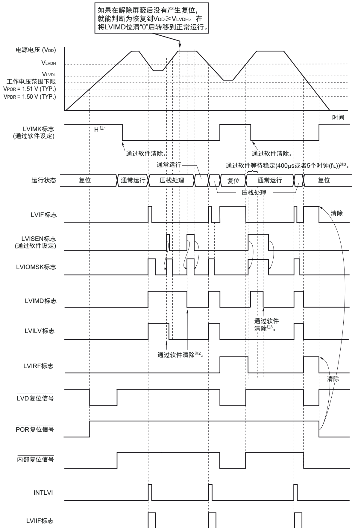
图 19-7 复位 & 中断信号的产生时序 (选项字节的 LVIMDS1、LVIMDS0=1、0) (1/2)
