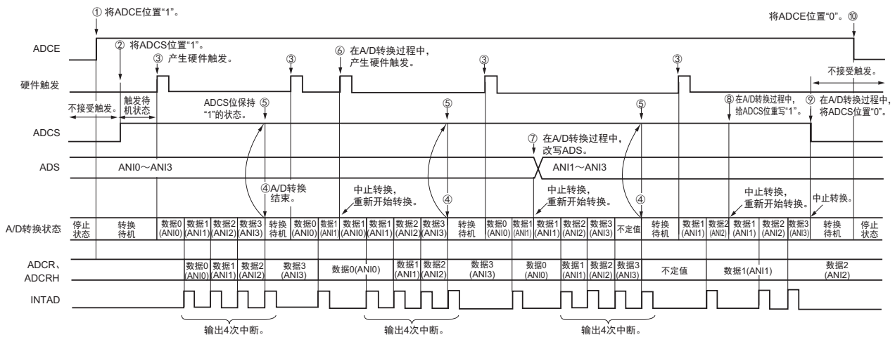
图 10-24 硬件触发无等待模式（扫描模式、单次转换模式）的运行时序例子
