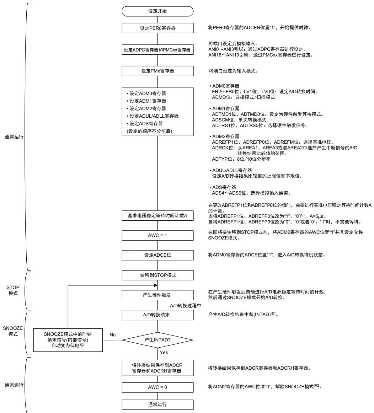
图 10-37 SNOOZE 模式的设定流程
