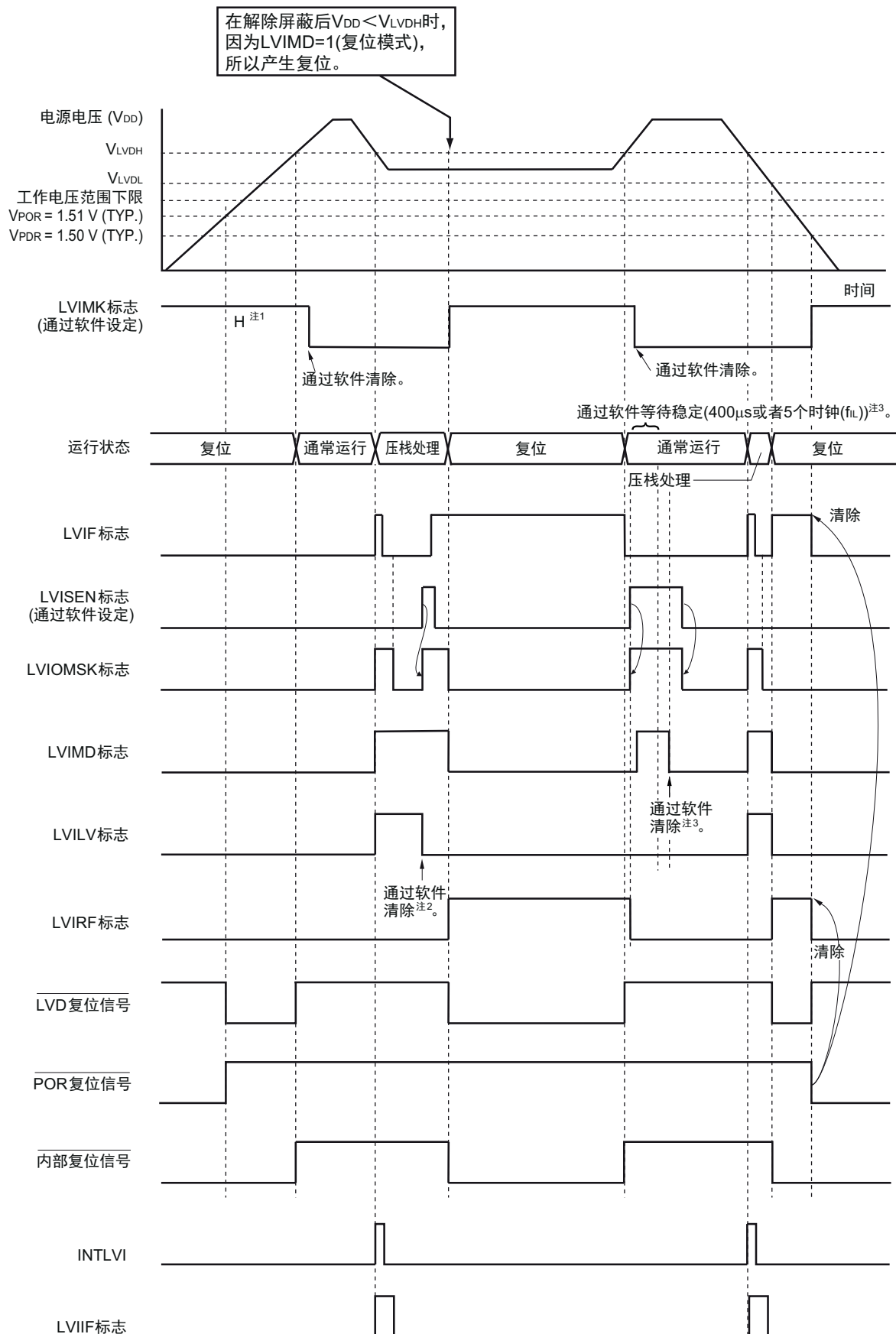
图 19-7 中断 &amp; 复位信号的产生时序 (选项字节的 LVIMDS1、LVIMDS0=1、0) (2/2)
