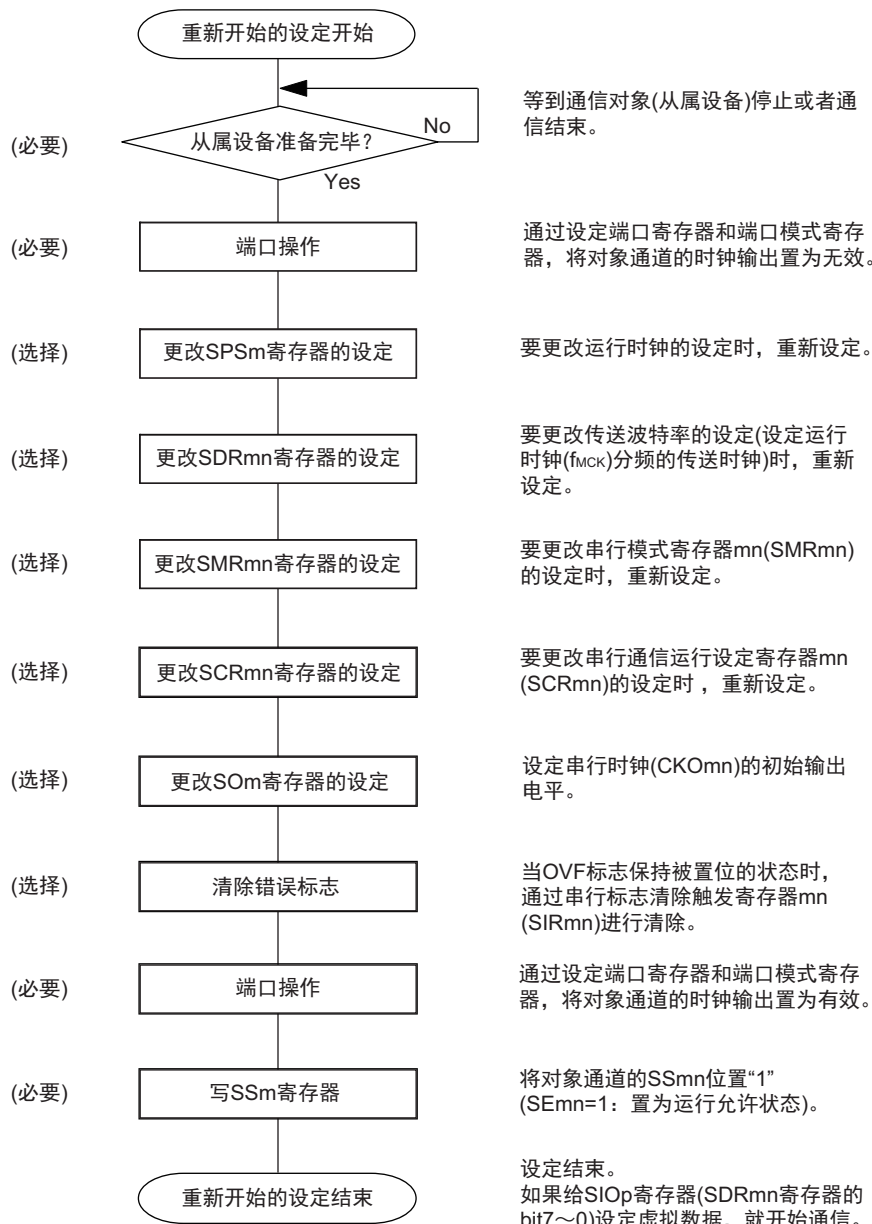
图 11-35 重新开始主控接收的设定步骤
