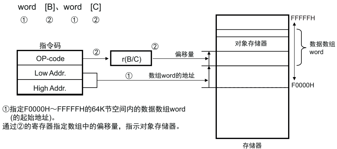
图 3-27 word[BC] 的例子
