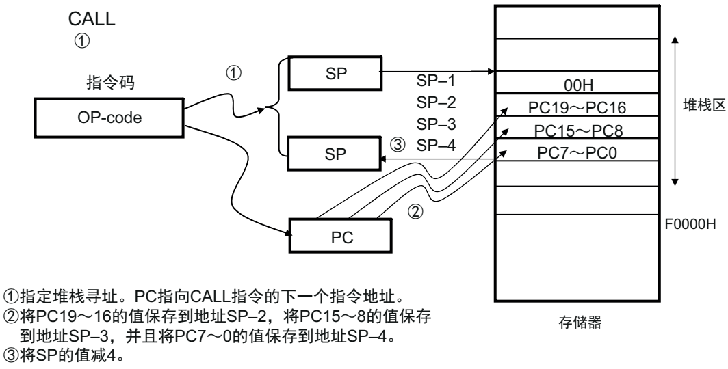
图 3-35 CALL、CALLT 的例子
