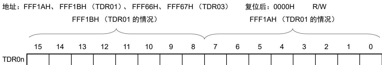
图 6-5 定时器数据寄存器 01、03 (TDR01、TDR03) 的格式
