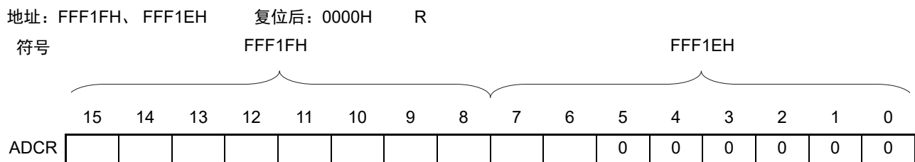
图 10-9 10 位 A/D 转换结果寄存器 (ADCR) 的格式
