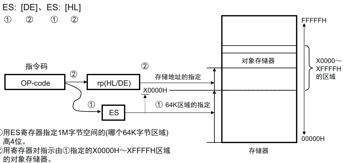
图 3-23 ES:[DE]、ES:[HL] 的例子
