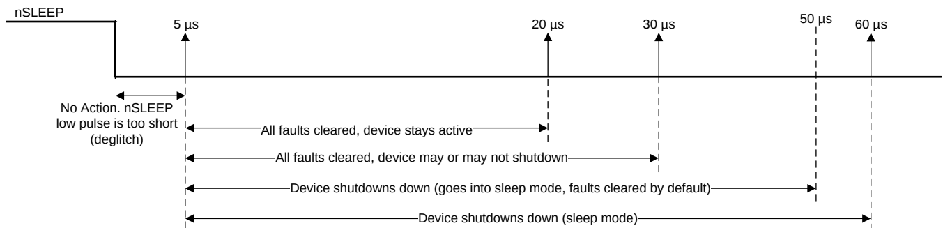
图 21. nSLEEP Reset Pulse
