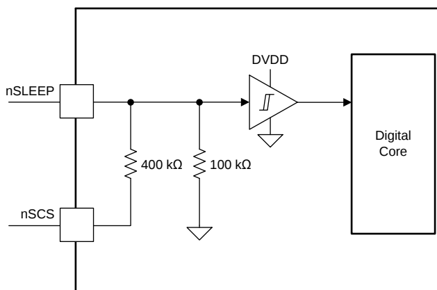
图 18. nSCS and nSLEEP Circuit
