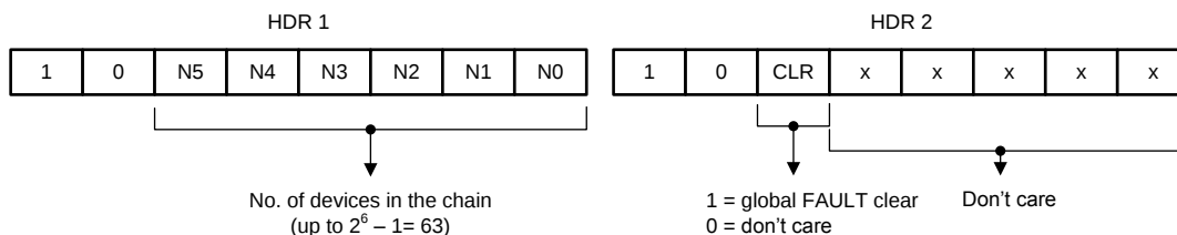
图 27. Header Bytes
