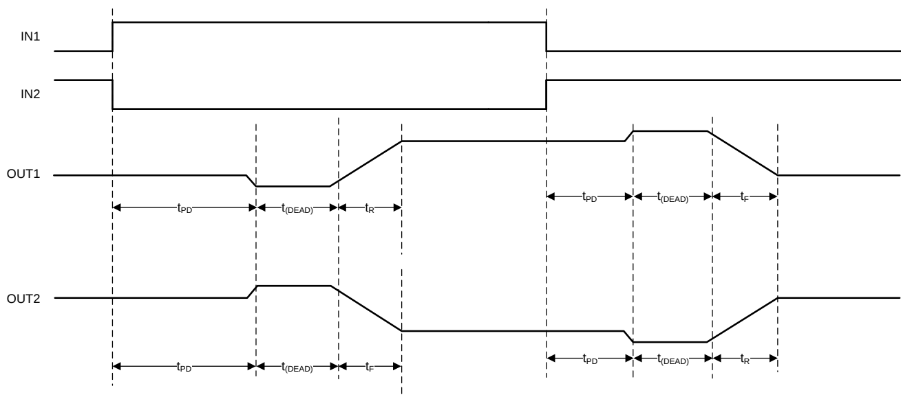
图 16. Propagation Delay Time
