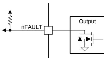
图 17. nFAULT Pin
