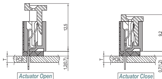
PCB ASS'Y
