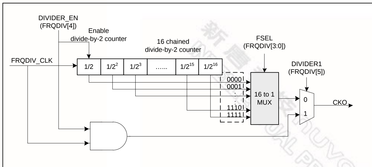
图 6-9 分频器框图
