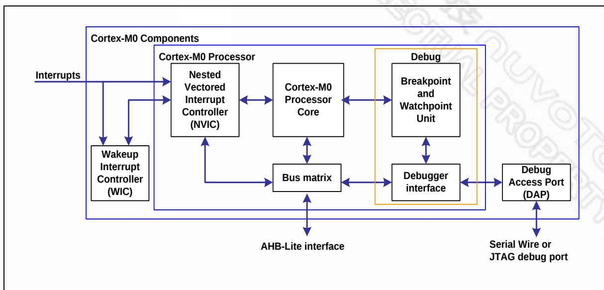
图6-1 功能框图
