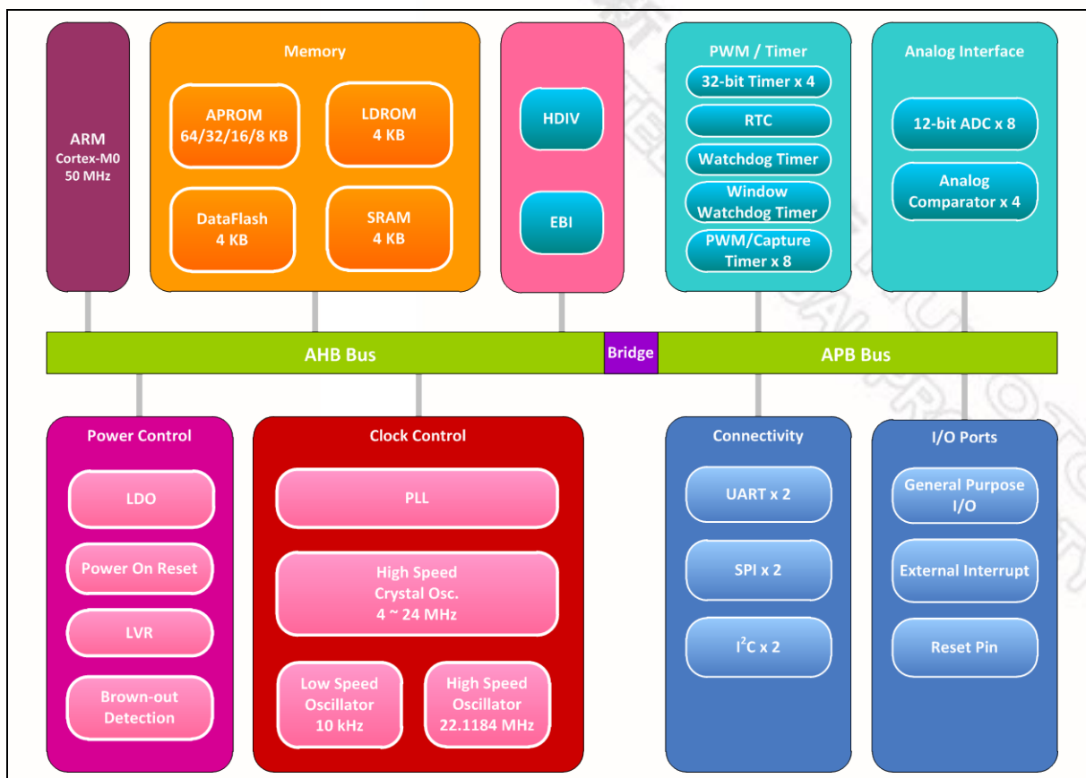
图 4-1 NuMicro™ M051 DN/DE 系列方块图
